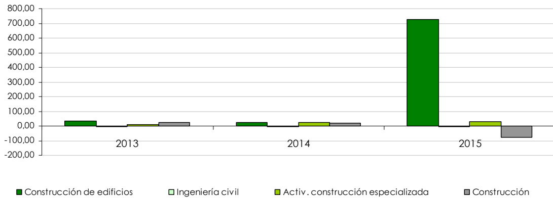
Gráfico 3.1 EBE sobre VAB coste de los factores Unidades: %
